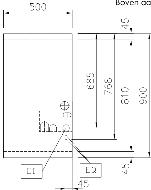
Boven aanzicht
